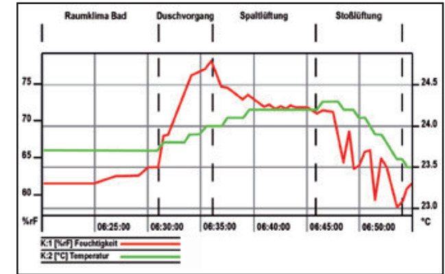
Originalausdruck Datenlogger
